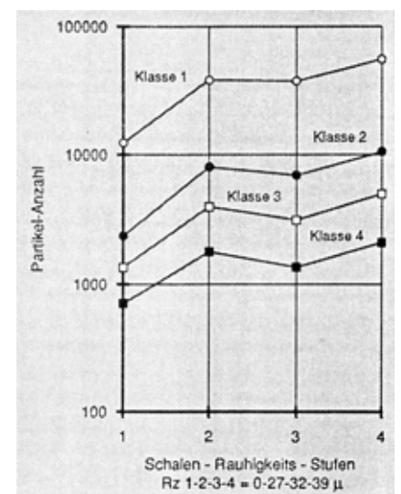
Abb. 11 Beispiel Cellulose-Polyester-Vlies Partikelfreisetzung, abgestuft nach 4 verschiedenen Klassenbreiten der Partikelgröße und 4 zunehmenden Stufen der Rauigkeit des Schalenbodens.
