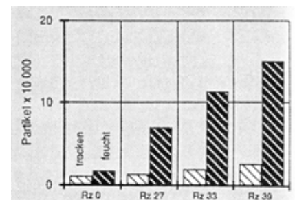
Abb. 9 Partikelfreisetzung > 0,19 µ von einem Viskose-Vlies, Vergleich feuchtes und trockenes Material
